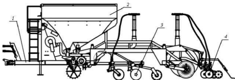
Рисунок – Схема почвообрабатывающе-посевного агрегата шириной захвата 9 метров
