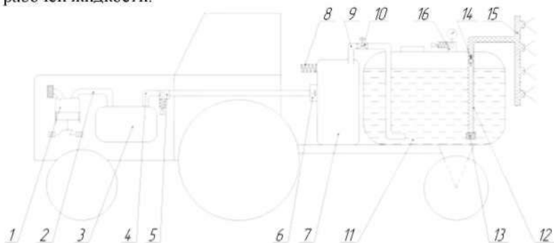
Рисунок – Схема опрыскивателя пневматического
