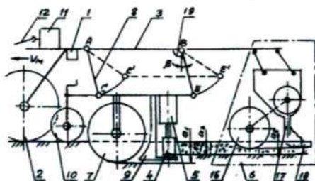
Рисунок – Электрифицированная машина для полосного подсева семян трав в дернину
