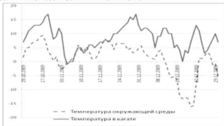
Рисунок – Изменение температуры воздуха в кагате в зависимости от температуры окружающей среды
